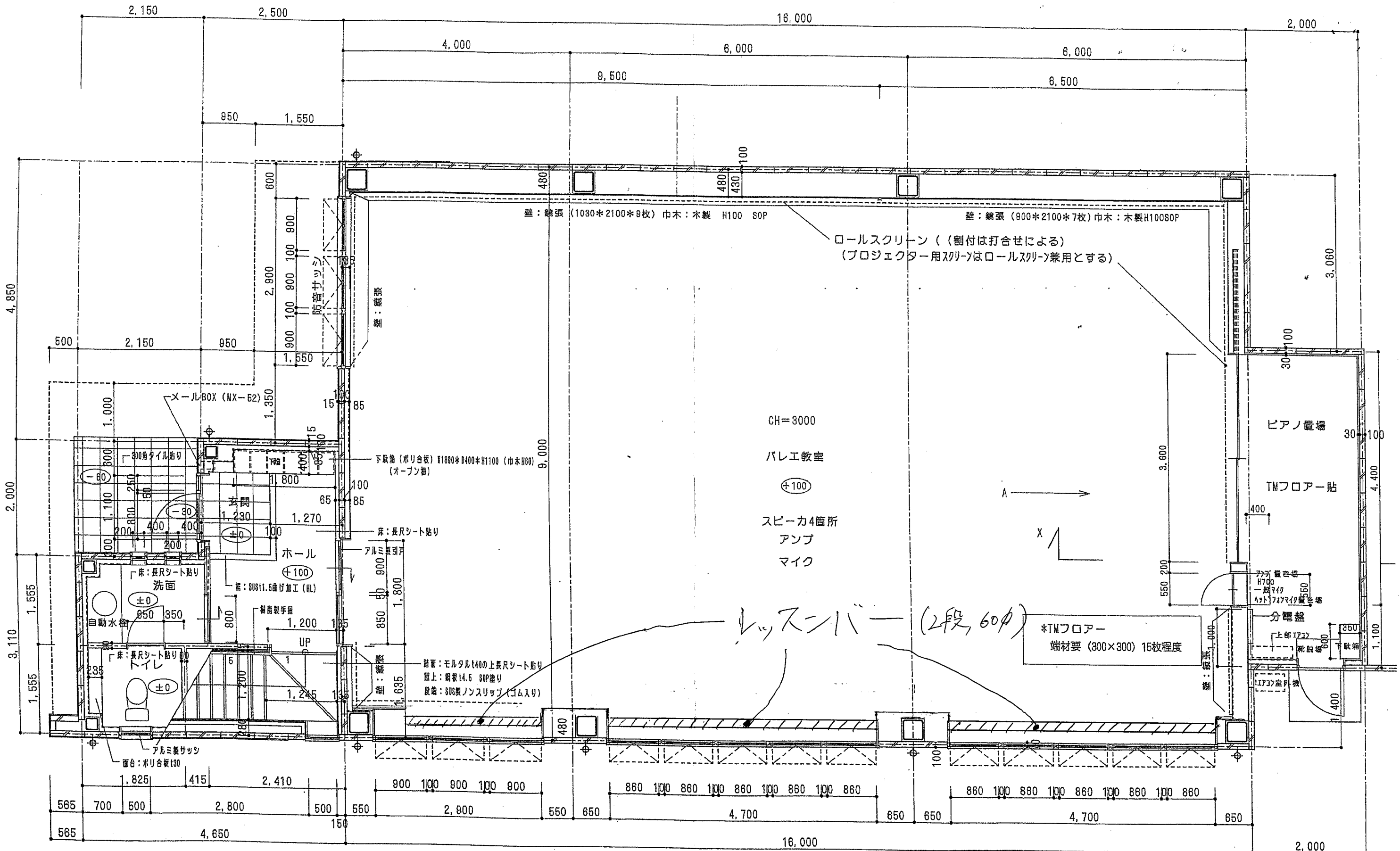
屋内階段 (2)、バレエ教室 1階平面詳細図 1/60
